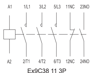
Scheme de conexiune
