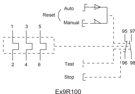
Schema de conexiune
